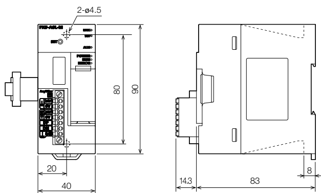
FX5-ASL-M
